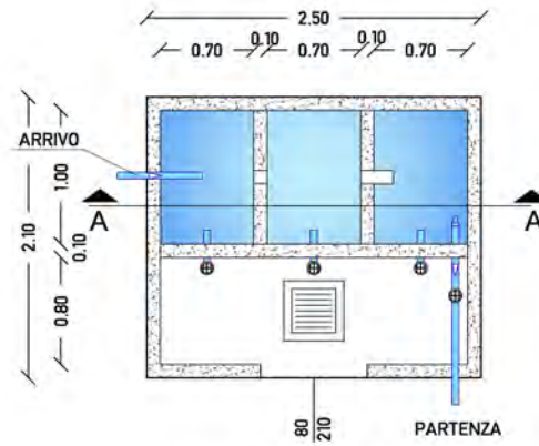
PIANTA
