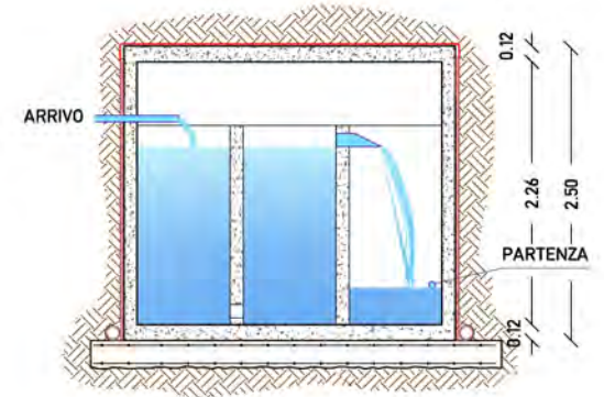
SEZIONE A-A'
